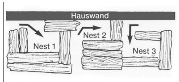
Abb. 13: Grundriss des Unterbaus einer Holzbeige, unter der mit Balkenreststücken (Höhe mindestens 10 cm) ein Labyrinth geschaffen wurde. Die Hohlräume deckt man mit Brettern ab. Man kann auch ein stabiles Weinkistchen (Schlupfloch nicht vergessen!) mit in die Holzbeige einbauen.
