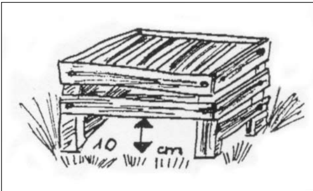
Abb. 15: Futterhaus aus einer umgedrehten Obstkiste. Auf das Dach nagelt man als Regenschutz eine Plastikfolie, besser noch Dachpappe.
