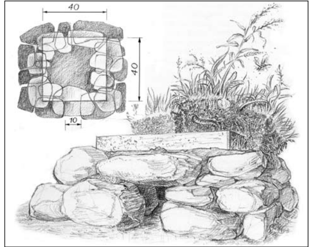
Abb. 8: Dieser Unterschlupf aus Natursteinen wird mit Erde und Grassoden bedeckt, so dass er von außen ganz zuwächst. Der etwa quadratische Innenraum hat eine Seitenlänge von 25 - 30 cm.
